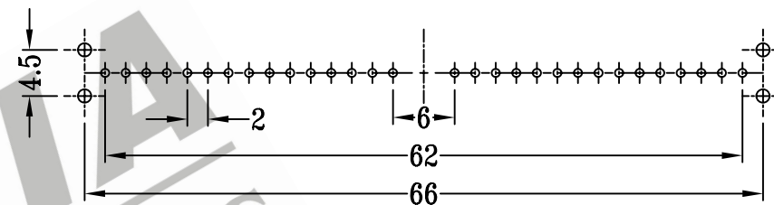
P.C.B LAYOUT
